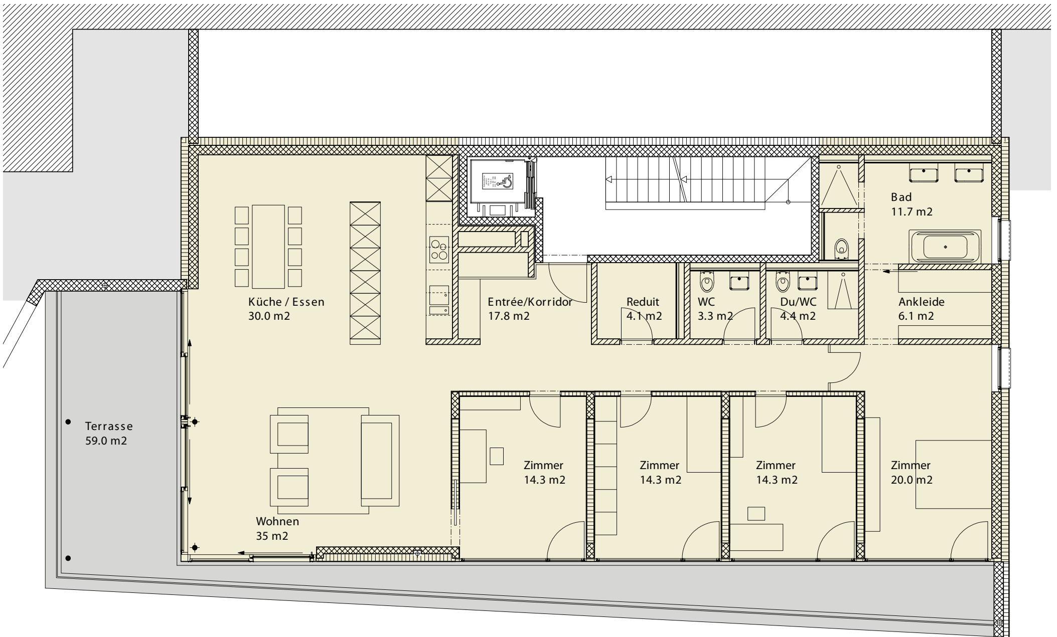
2. Obergeschoss Haus 21 BGF 215.2 m 2
